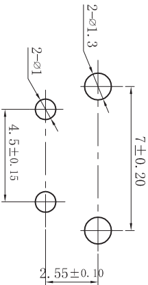
印制线路板 P.C.B layout
