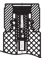
接頭剖面圖
