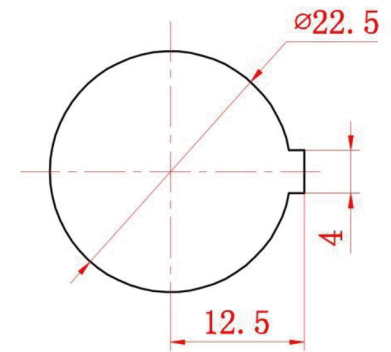
安装尺寸
